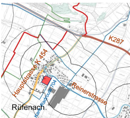
Abbildung 22: Verkehrsnetz Schlüsselgebiet Neumattweg, Rüfenach
